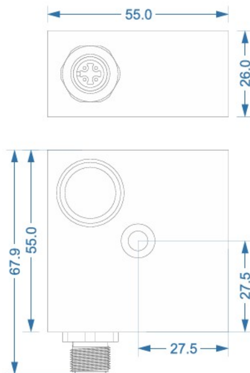
外形寸法図
