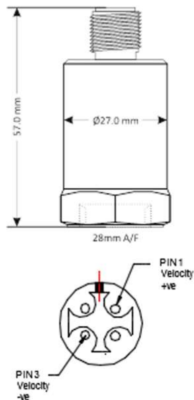
外形寸法図
