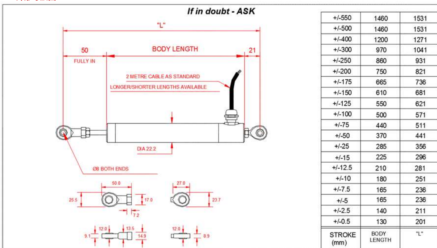
外形寸法図
