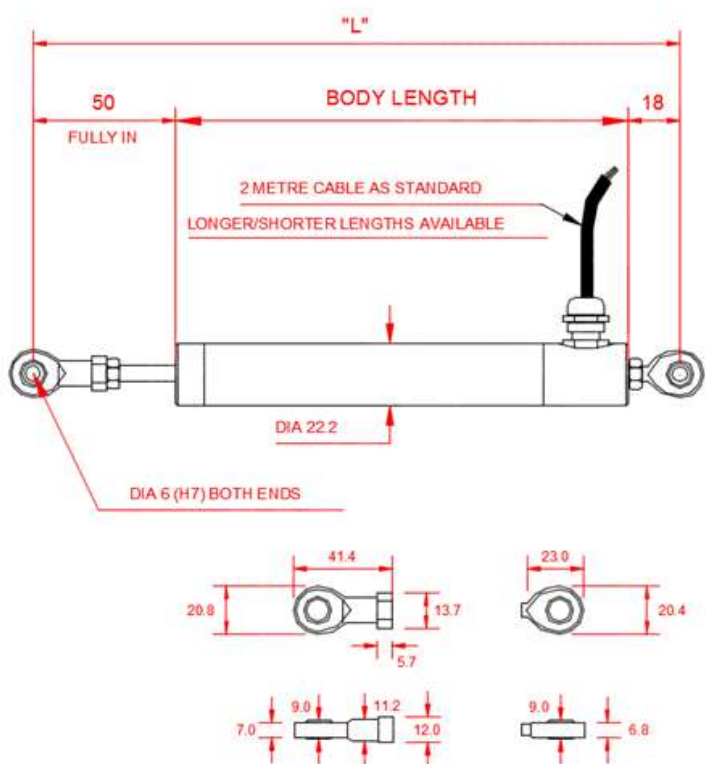
外形寸法図
