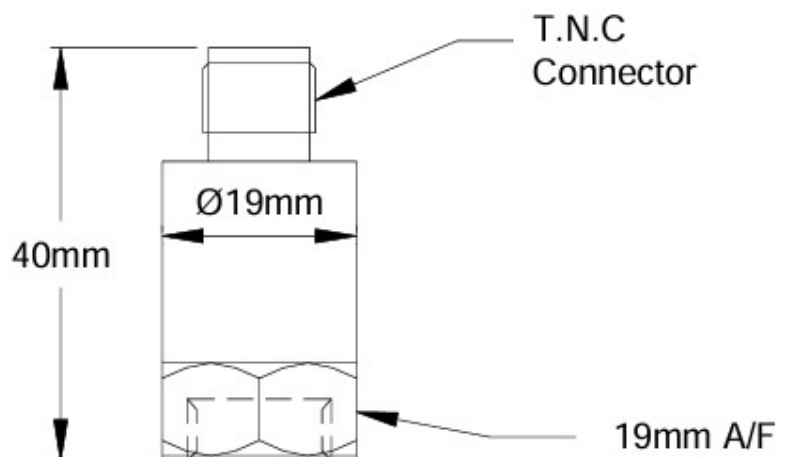
外形寸法図
