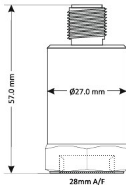
外形寸法図
