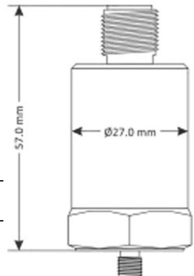
外形寸法図
