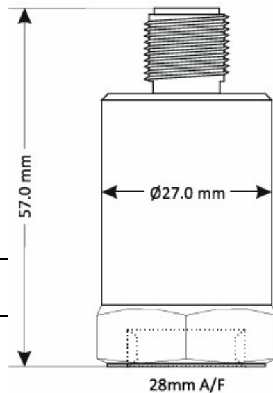
外形寸法図
