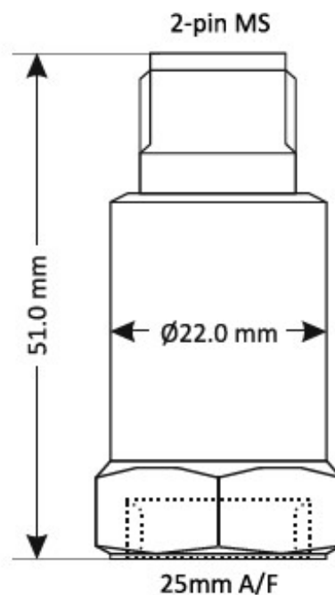
外形寸法図
