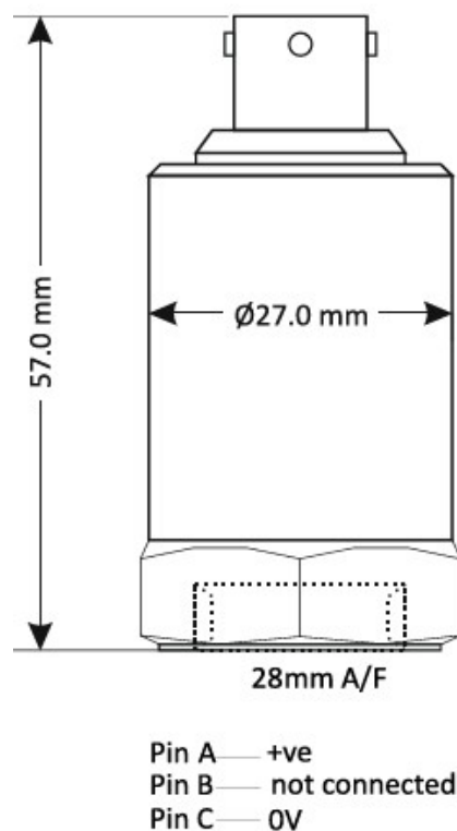
外形寸法図
