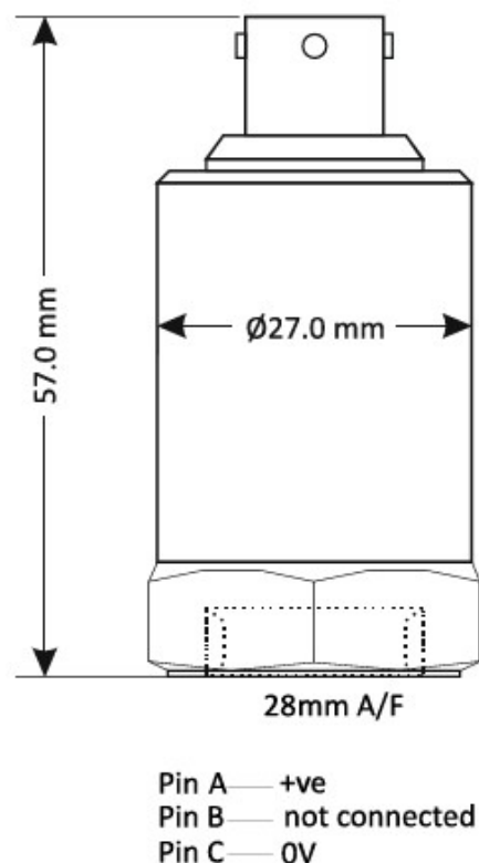
外形寸法図
