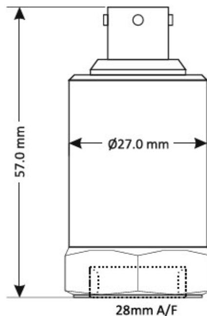
外形寸法図
