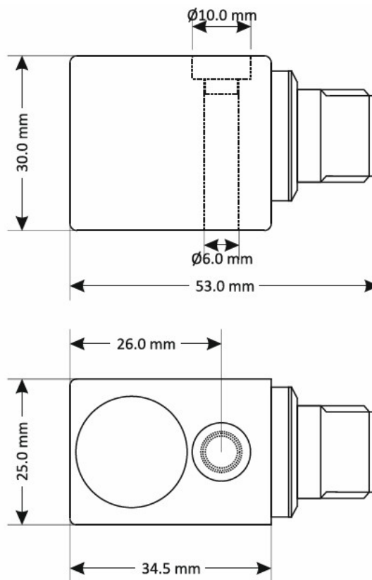
外形寸法図
